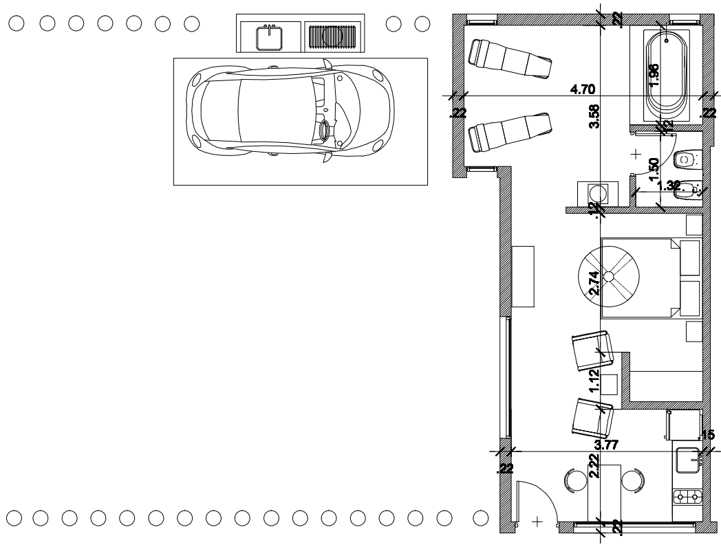
Planta Habitación Suite
